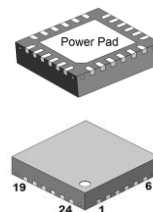
AS3330F QFN-24 4x4mm 0,5mm
